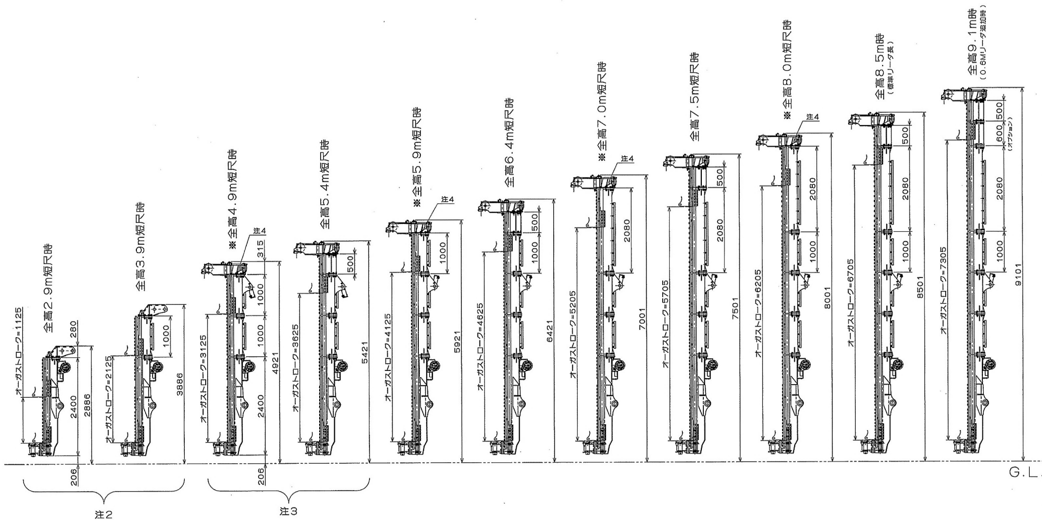
短尺フロント組図 F159 J64470参照
